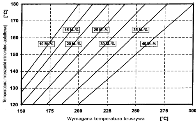
Tablica 13. Temperatura kruszywa w zależności od ilości zimnego i suchego granulatu asfaltowego
